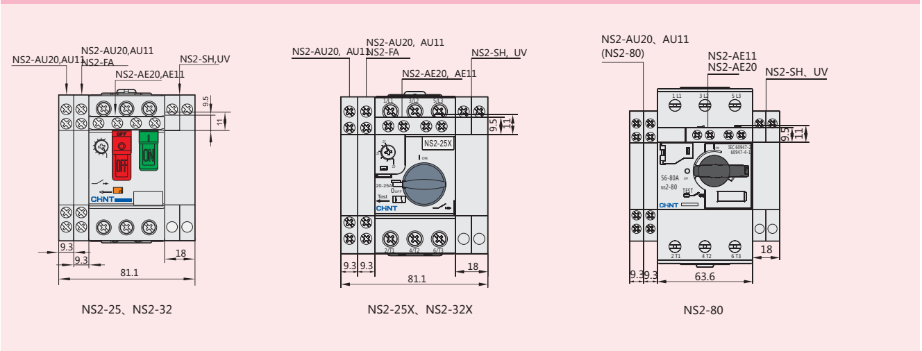
附件安装位置和安装尺寸
