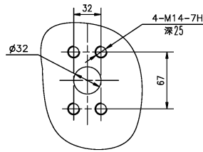
图 1 压料油缸接口尺寸
